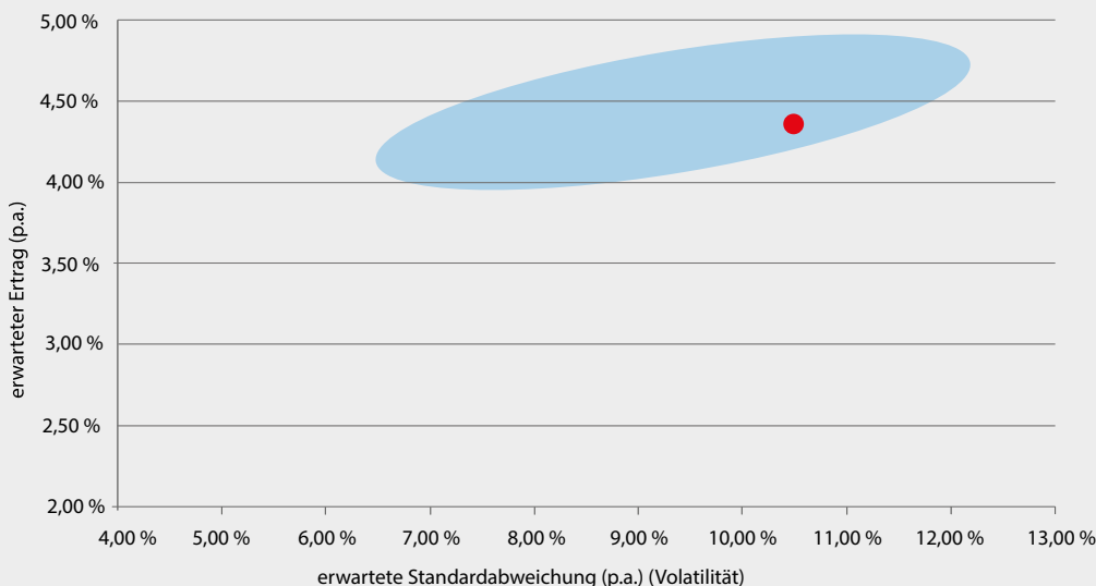
VRG 146 - Ertrag-Risikoprofil (Erwartung auf Basis der strategischen Asset Allocation, Stichtag 01.01.2023)
